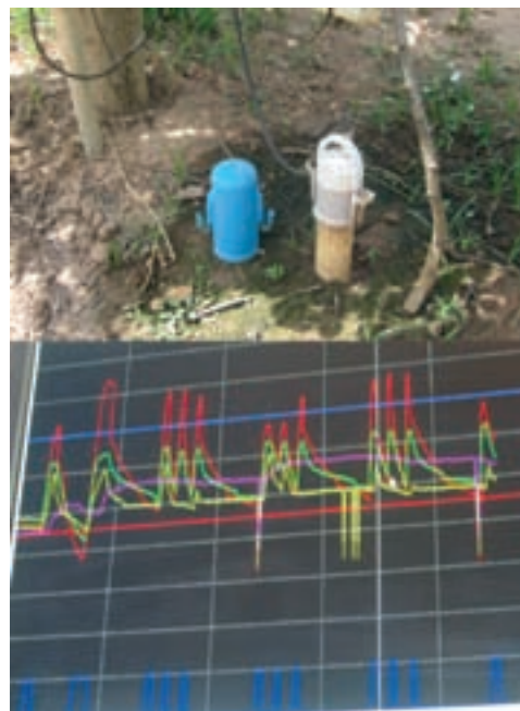
Sondas FDR que hacen la lectura de humedad en el suelo. Los datos recogidos a distintas profundidades se reflejan con varias gráficas en la pantalla del ordenador, desde donde se programa el riego.
